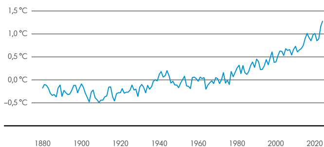
Globale Temperaturentwicklung (relativ zum Durchschnitt von 1951–1980)
